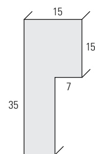
15.1810.35 LI
