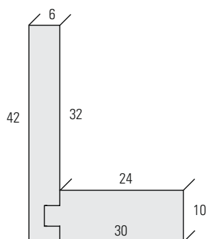
30.2202.42 EI 30.2202.42 LI
