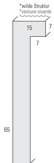
15.1825.65 LI
