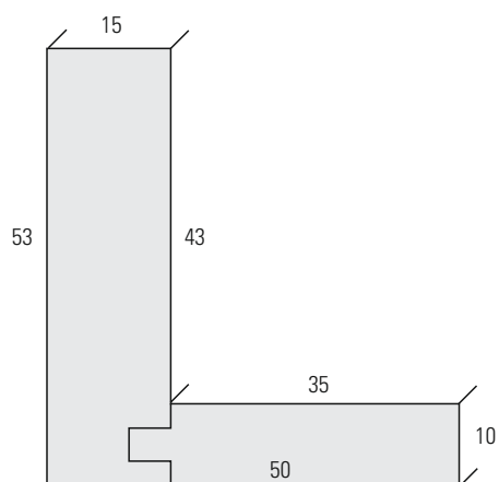
50.2205.53 LI
