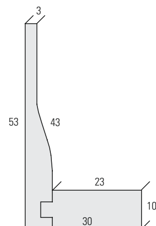
30.2207.53 EI 30.2207.53 LI
